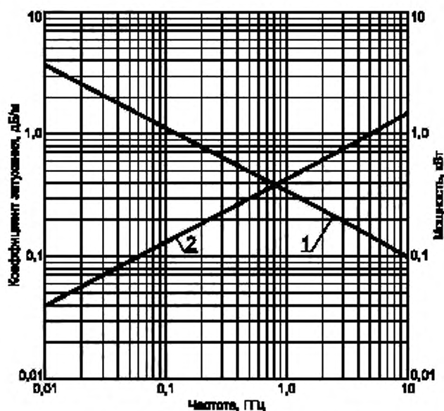
Частотные зависимости
